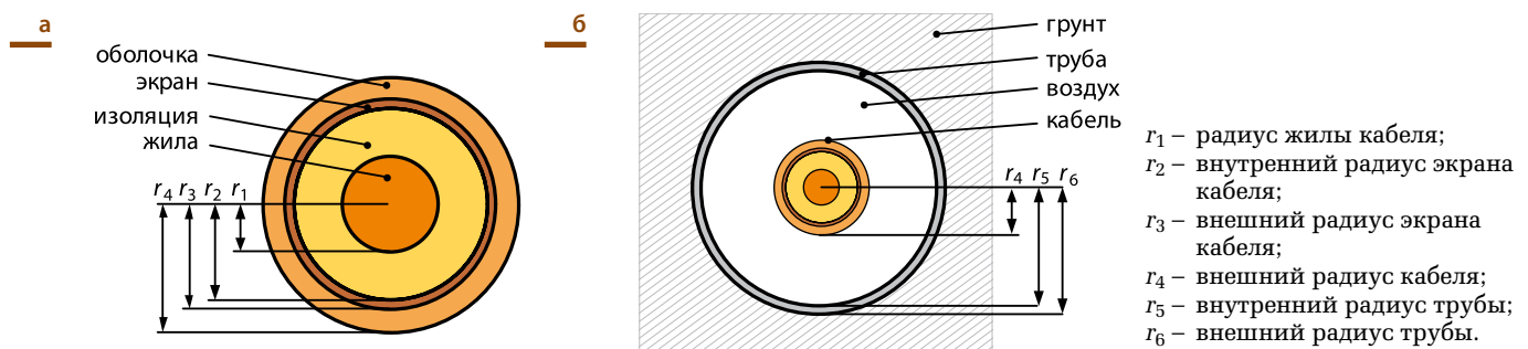
• Рис. 1. Силовой однофазный кабель, проложенный в полиэтиленовой трубе в грунте а) конструкция и параметры кабеля; б) способ прокладки и параметры трубы
