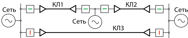
Сложная многоузловая схема сети, требующая расчета режимов Рис. 2 •
