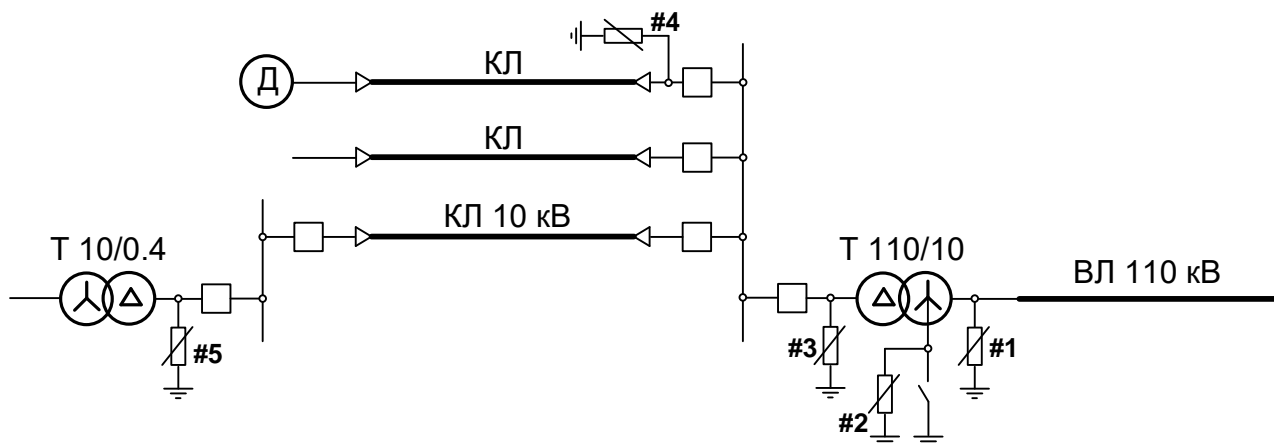
Пример №1. Схема электроснабжения предприятия.
