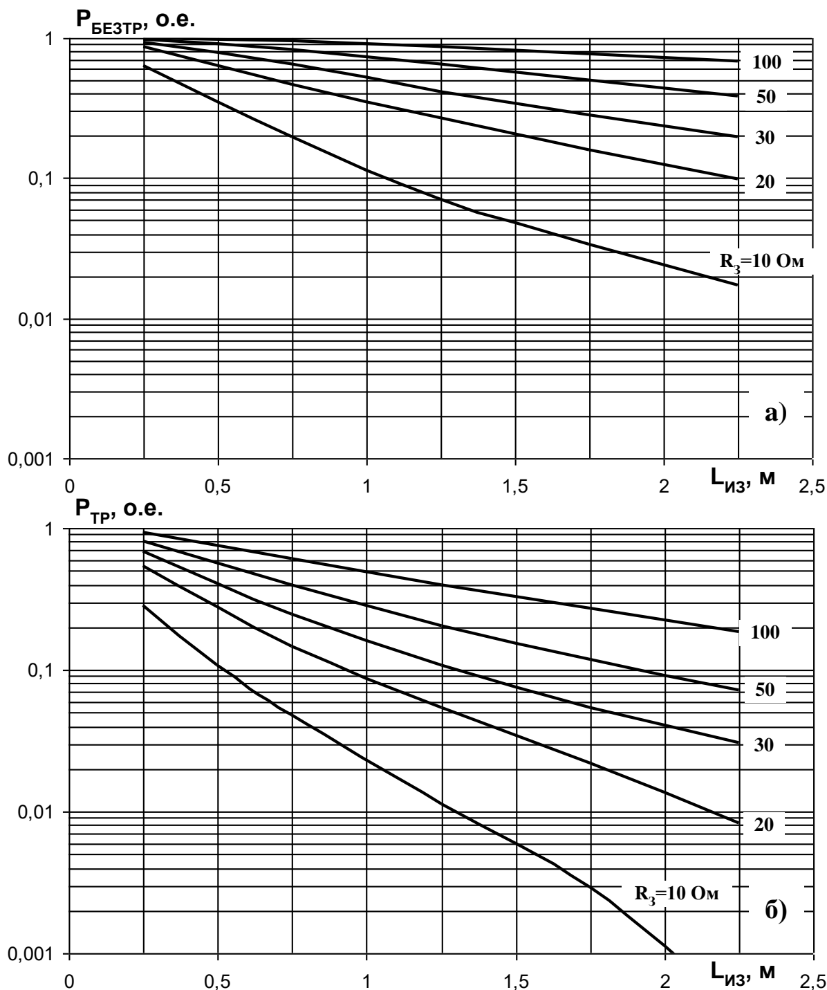
Рис.3.8. Вероятность перекрытия изоляции одноцепной ВЛ 110 кВ в зависимости от сопротивления заземления опор и длины гирлянды изоляторов: (а) – при разрядах молнии в опору линии без троса, (б) – при разрядах молнии в трос линии с тросом.
