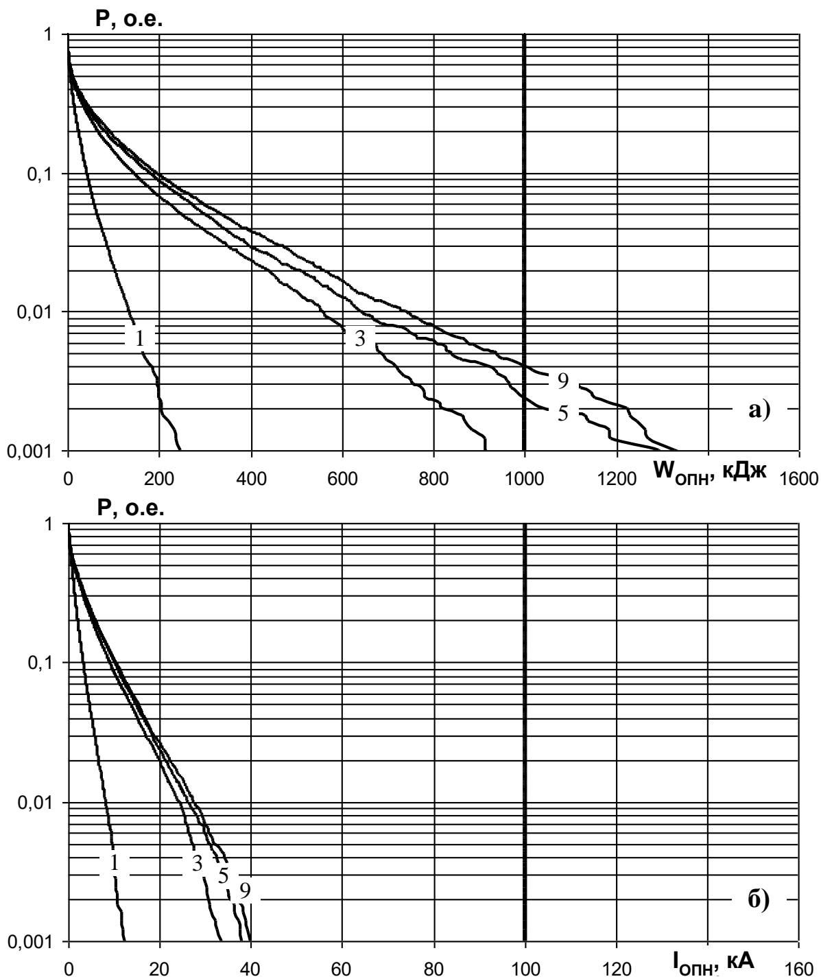
Рис.3.17. Энергия (а) и максимальное значение тока (б) в наиболее нагруженном ОПН при разряде молнии в опору одноцепной ВЛ 110 кВ без троса в зависимости от числа моделируемых опор: 1, 3, 5, 9. Рассмотрен случай: R_3 = 30 Ом, три ОПН на каждой опоре.
