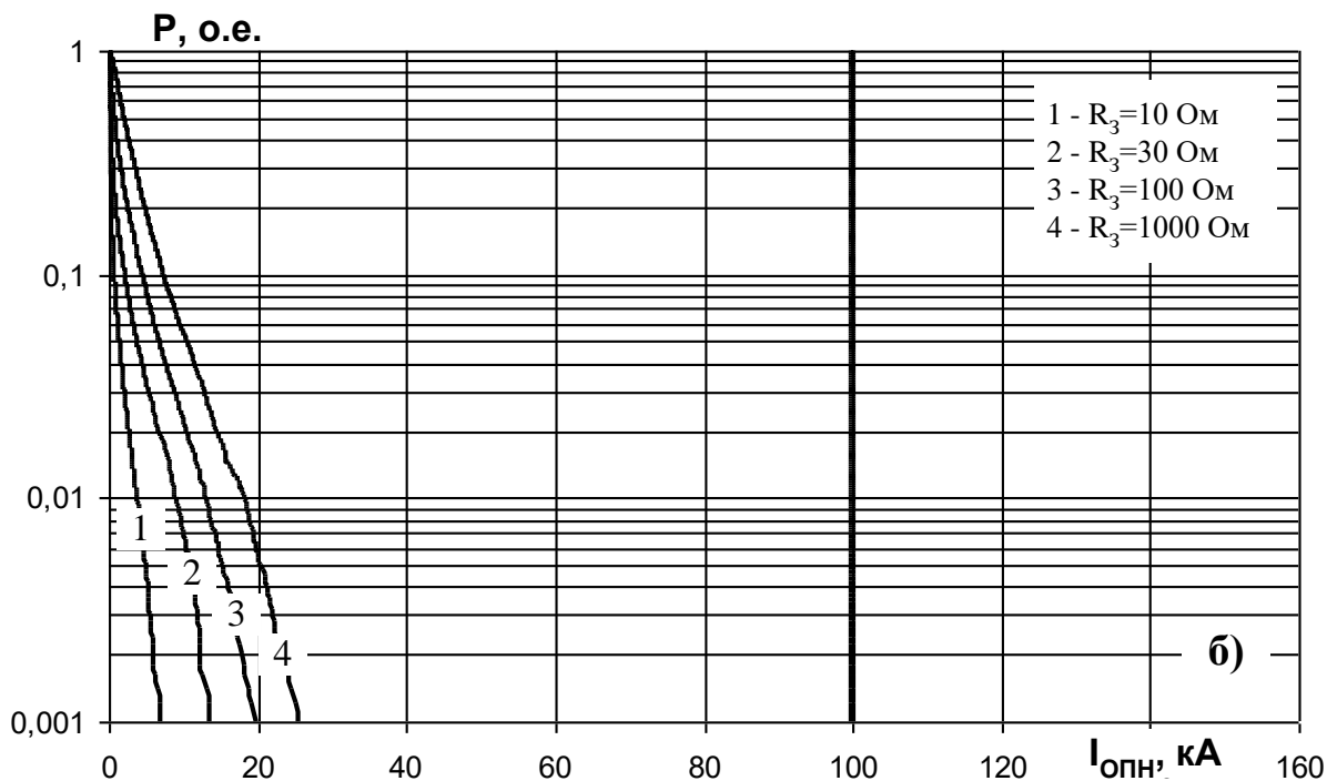
Рис.3.20. Энергия, выделяющаяся в наиболее нагруженном ОПН при разряде молнии в трос одноцепной ВЛ 110 кВ (три ОПН на каждой опоре).
