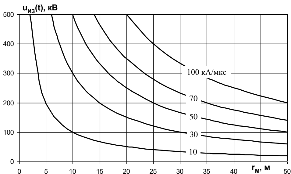
Рис.1.18. Индуцированное напряжение на изоляции ВЛ в зависимости от удаленности места разряда молнии и скорости изменения тока молнии (кА/мкс).
