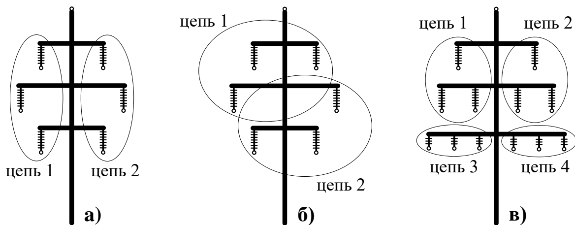
Рис.1.20. Варианты размещения цепей на различных многоцепных опорах.
